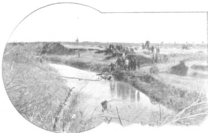
Наводка мостика на притокъ р. Шахе.
