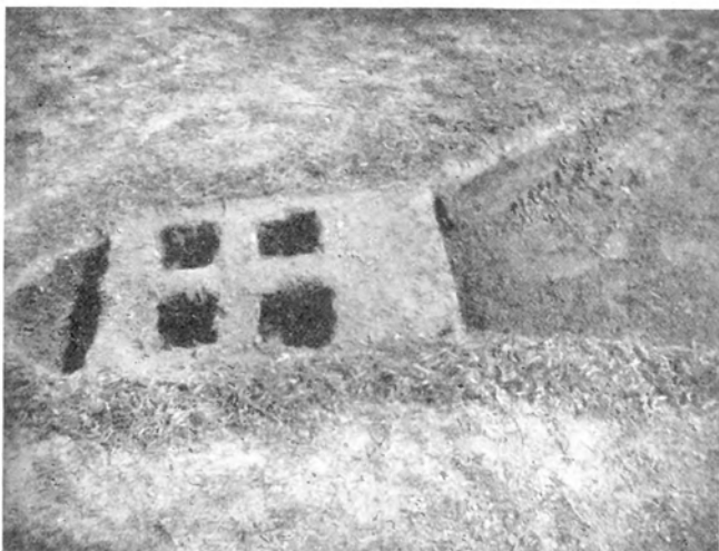
Очаги капитана фонъ-Рентель для солдатскихъ котелковъ (примѣнявшіеся на войнѣ 1904—1905 г.).
